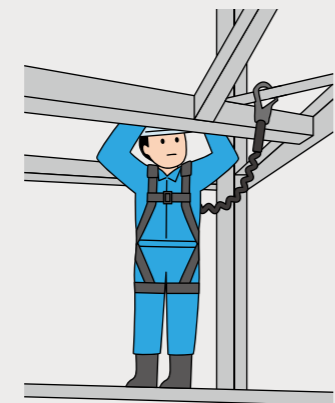
フルハーネス型(一本つり)
