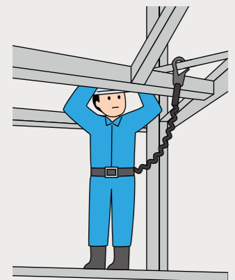
胴ベルト型(一本つり)
