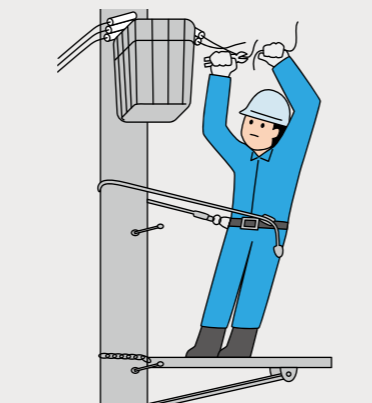
胴ベルト型(U字つり)
