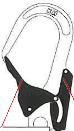
外れ防止レバー
